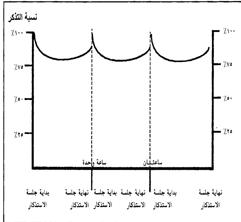
شكل رقم ٥ منحنى التذكر ب.
